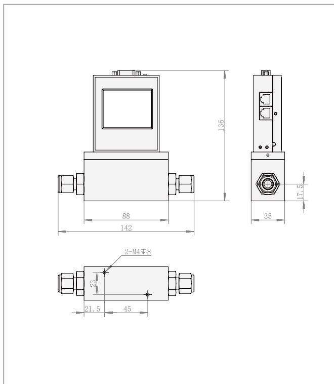
▲ ACU30FC-MM 高精度差压式流量计
