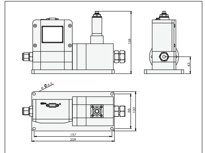
▲ ACU20FE-XC 科里奥利质量流量控制器
