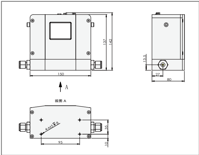
▲ ACU20FE-BM 科里奥利质量流量计
