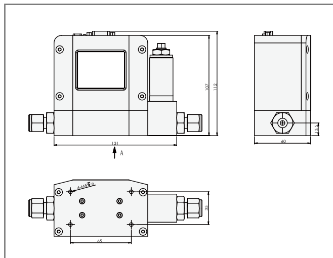
▲ ACU20FE-LC 科里奥利质量流量控制器
