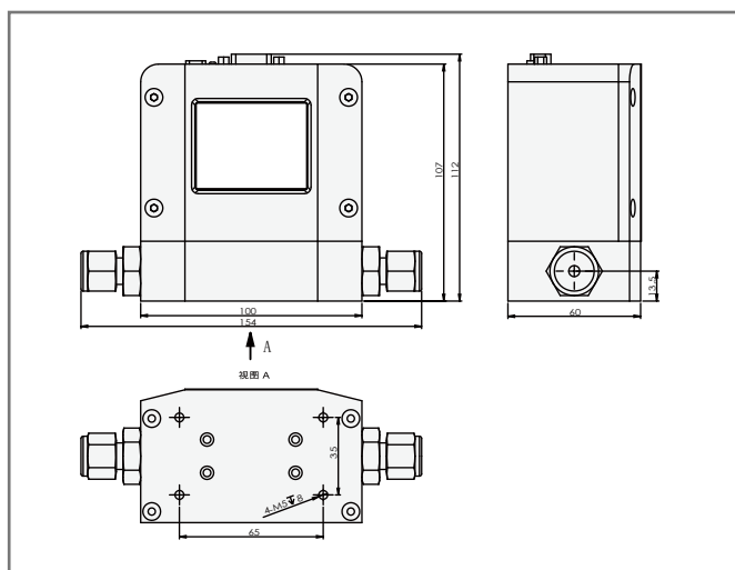
▲ ACU20FE-MM 科里奥利质量流量计
