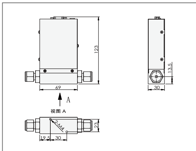
▲ ACU20FE-SM 科里奥利质量流量计
