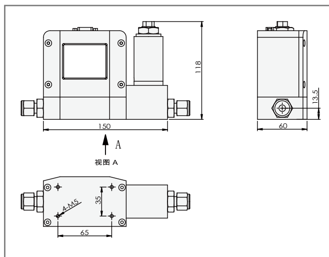
▲ ACU20FE-MC 科里奥利质量流量控制器
