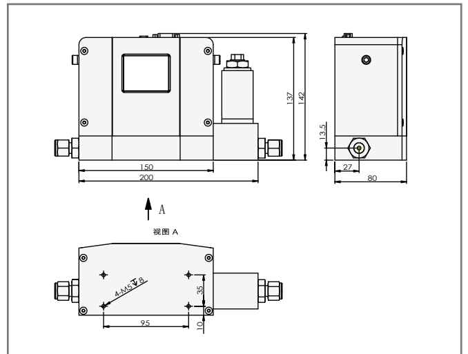
▲ ACU20FE-BC 科里奥利质量流量控制器
