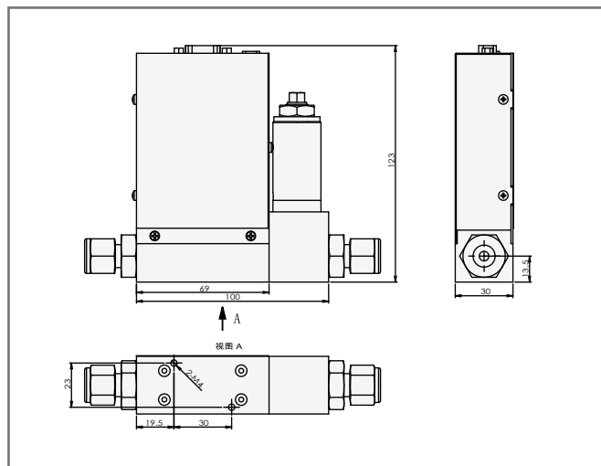
▲ ACU20FE-SC 科里奥利质量流量控制器
