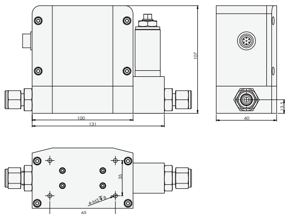
▲ ACU20FEH-LC质量流量控制器部分尺寸图
