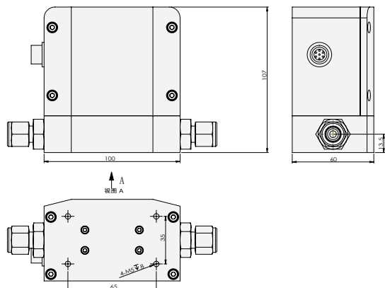
▲ ACU20FEH-MM质量流量计部分尺寸图
