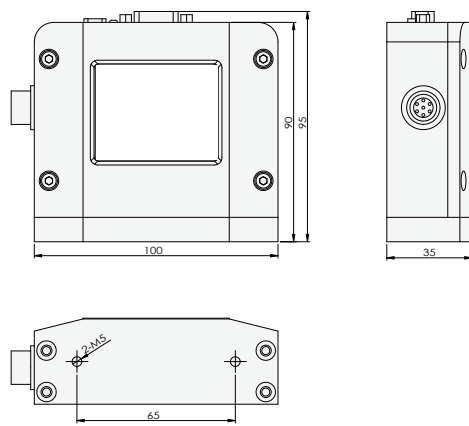
▲ ACU20FEH电气部分尺寸图
