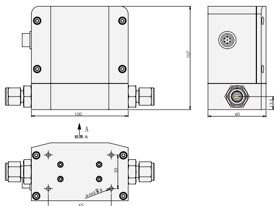
▲ ACU20FEH-XM质量流量计部分尺寸图
