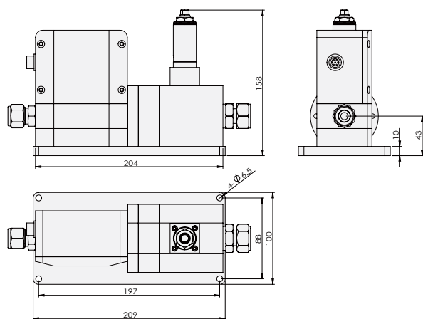
▲ ACU20FEH-XC质量流量控制器部分尺寸图
