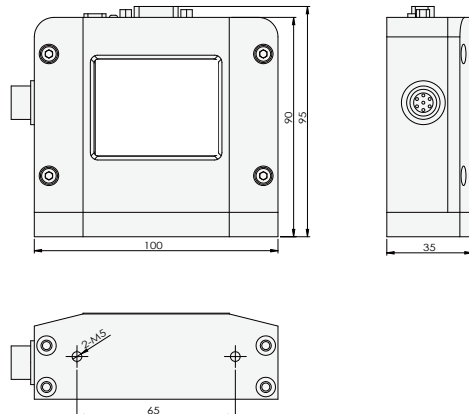
▲ ACU20FEH电气部分尺寸图
