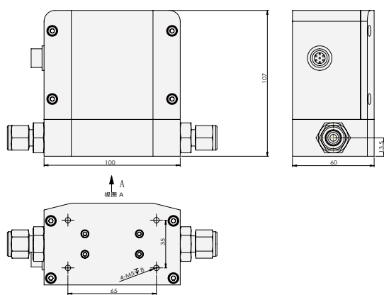
▲ ACU20FEH-LM质量流量计部分尺寸图
