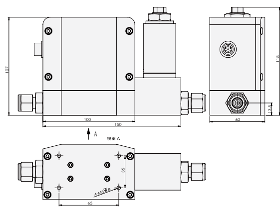
▲ ACU20FEH-MC质量流量控制器部分尺寸图
